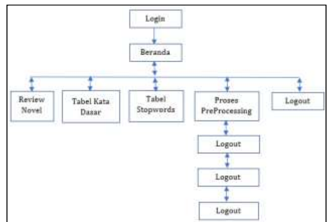
Gambar 4. Struktur Navigasi Aplikasi
