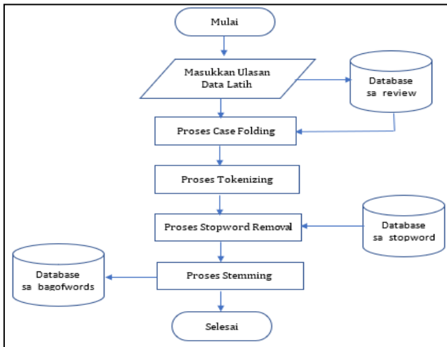
Gambar 3. Flowchart Pembentukan Data Latih
